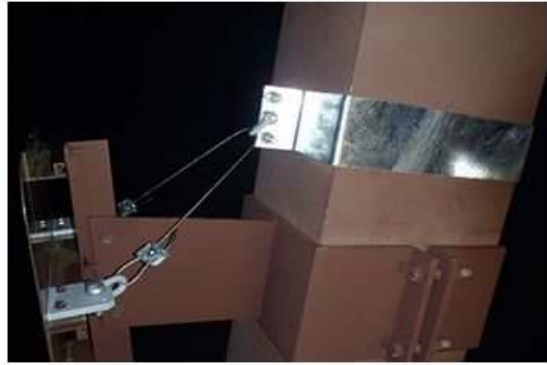
標識板落下防止対策
